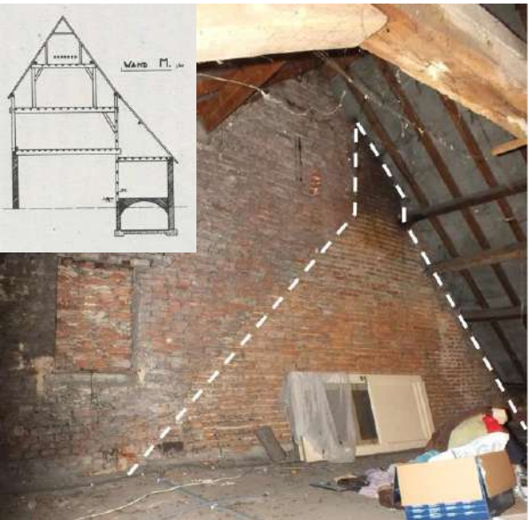
afb. 35: Zolder, scheidsmuur met bouwsporen van vroegere volume bedaking naar typologie van Kempisch woonhuis.
