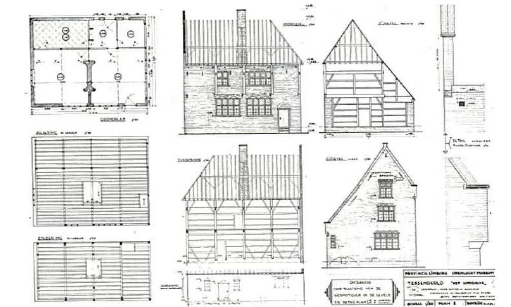
afb. 24: Tessenderloo. Het hooghuis. Plan voor de herbouw in Bokrijk. 21 augustus 1971 © Bron: H. Ruhe, Het dorpswoonhuis in de Kempen vanaf de vijftiende tot de negentiende eeuw, Zaltbommel, 1980: 149.
