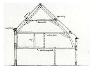
afb. 21: Typeplan en dwarsnede ©H. Ruhe, bewerkt door ARAT architecten.
