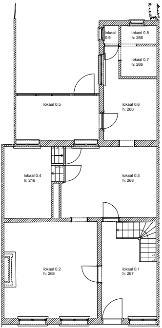
afb. 26: Grondplan © ARAT architecten.
