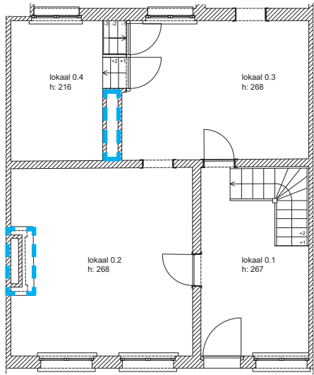
afb. 34: Grondplan © ARAT architecten.
