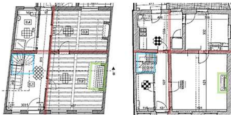
afb. 20: Grondplan gelijkvloerse verdieping 54 (links) en 78 (rechts) © ARAT architecten.
