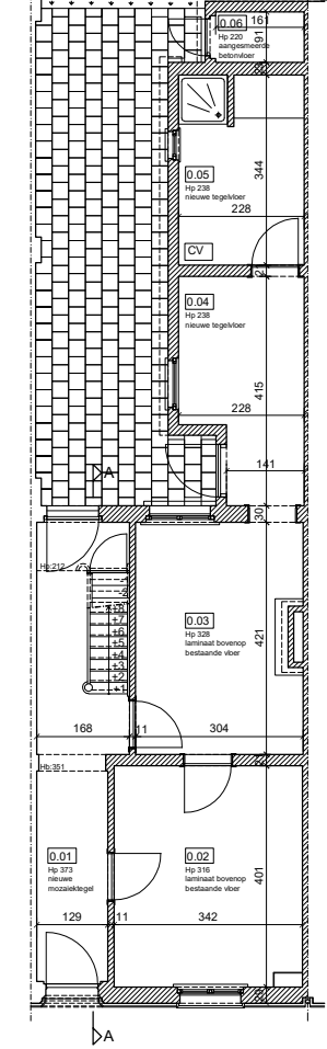
GRONDPLAN
